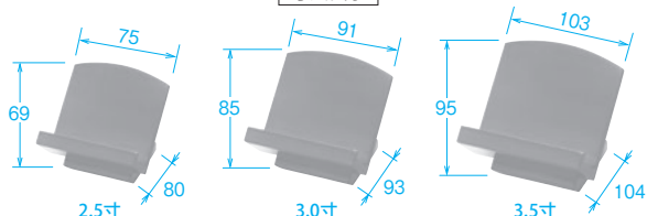
寸法表示
