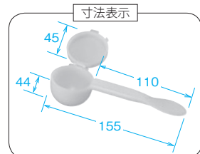
寸法表示
