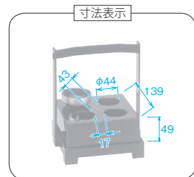
寸法表示
