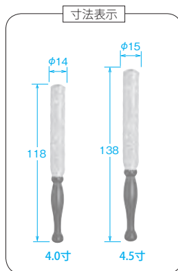
寸法表示
