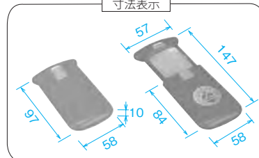
寸法表示
