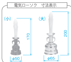
電気ローソク 寸法表示
